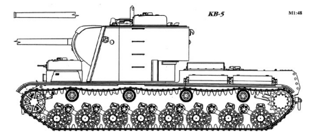
KB-5, вид сбоку («Бронеколлекция», №1, 2002)
